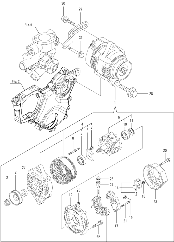
Fig.15. GENERATOR
